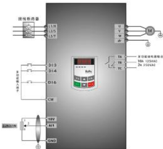
图 5-9 接线图 3
