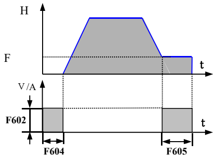
图 6-20 直流制动
