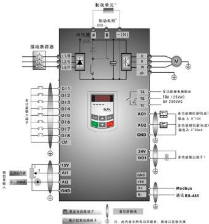
图 4-11 三相变频器标准配线图 (NPN 方式)
