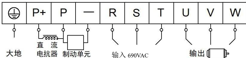
图 4-2 接线示意图
